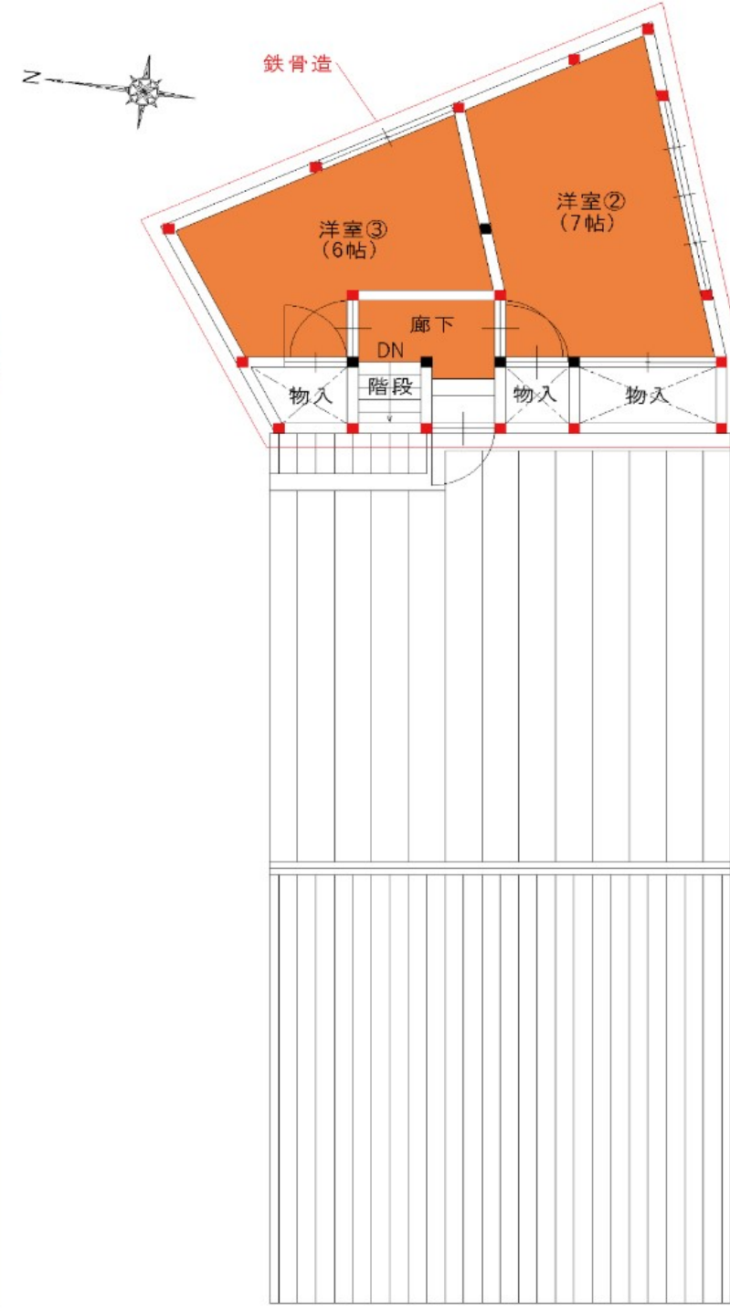
3階平面図
