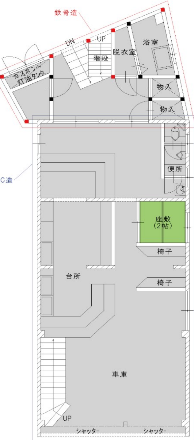
1階平面図
