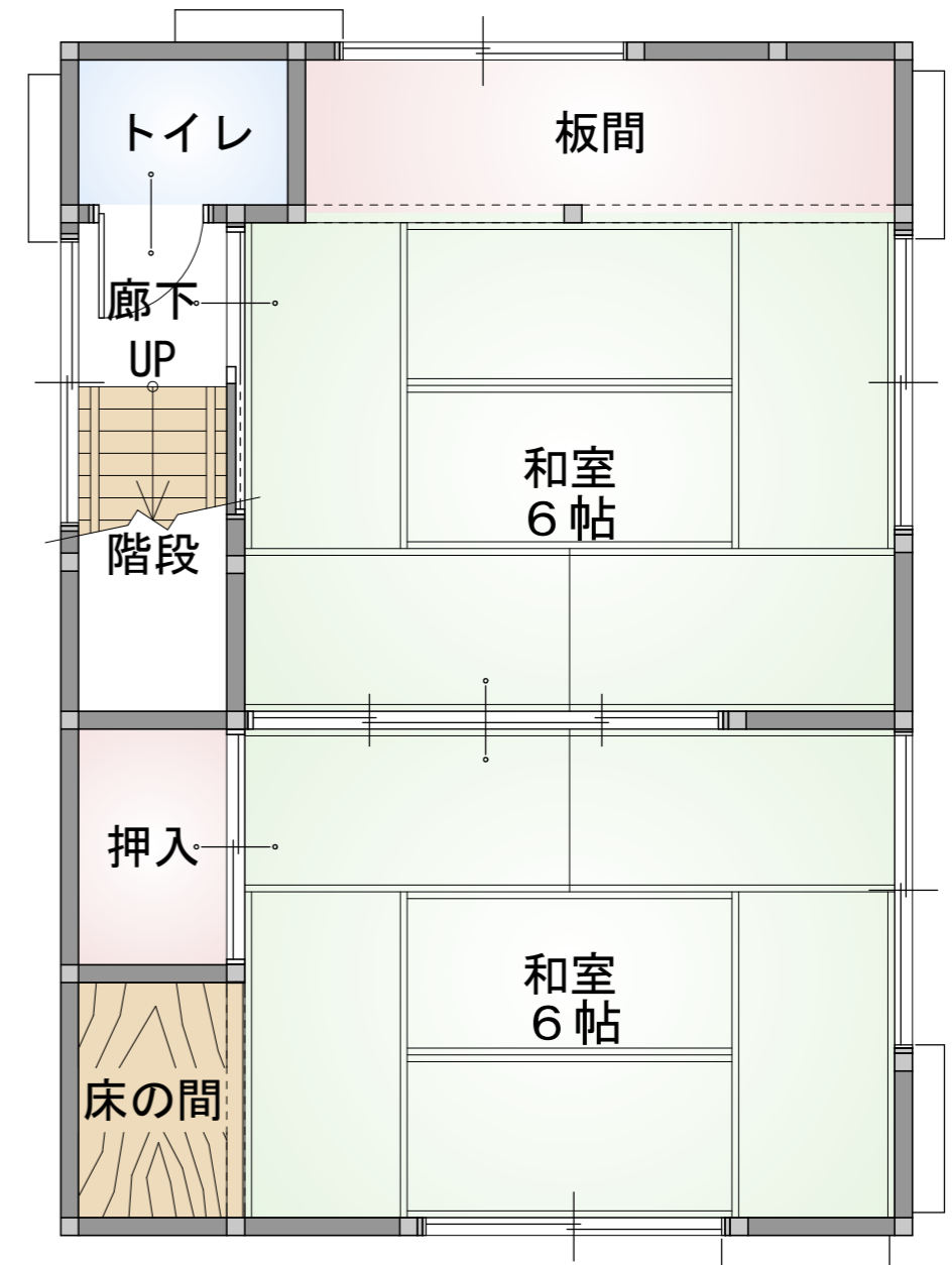
2階
