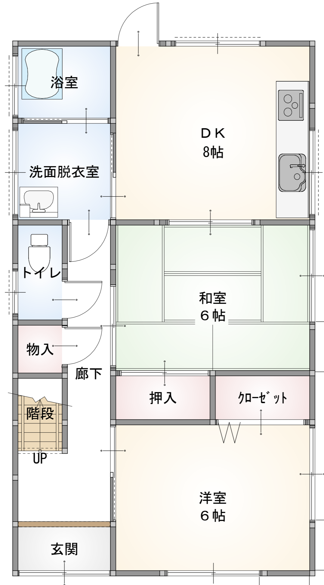
1階
